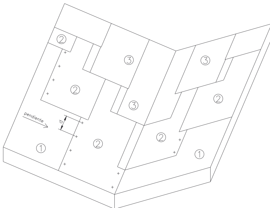
Figure 6 Noue de pente nulle
